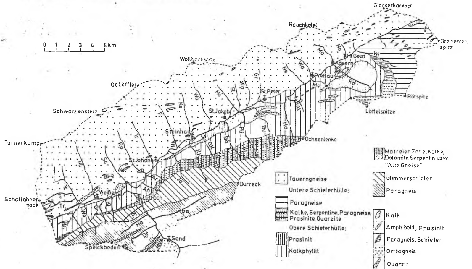
Geologische Skizze des Ahrntales (aus Chr. Hannß 1967)
